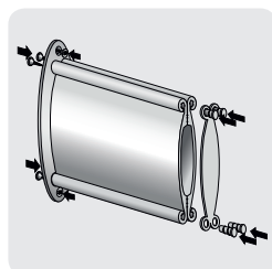
Haakse montage
